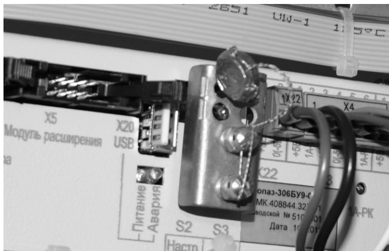
Рисунок В.2 Пломбировка фиксирующей планки блока управления
