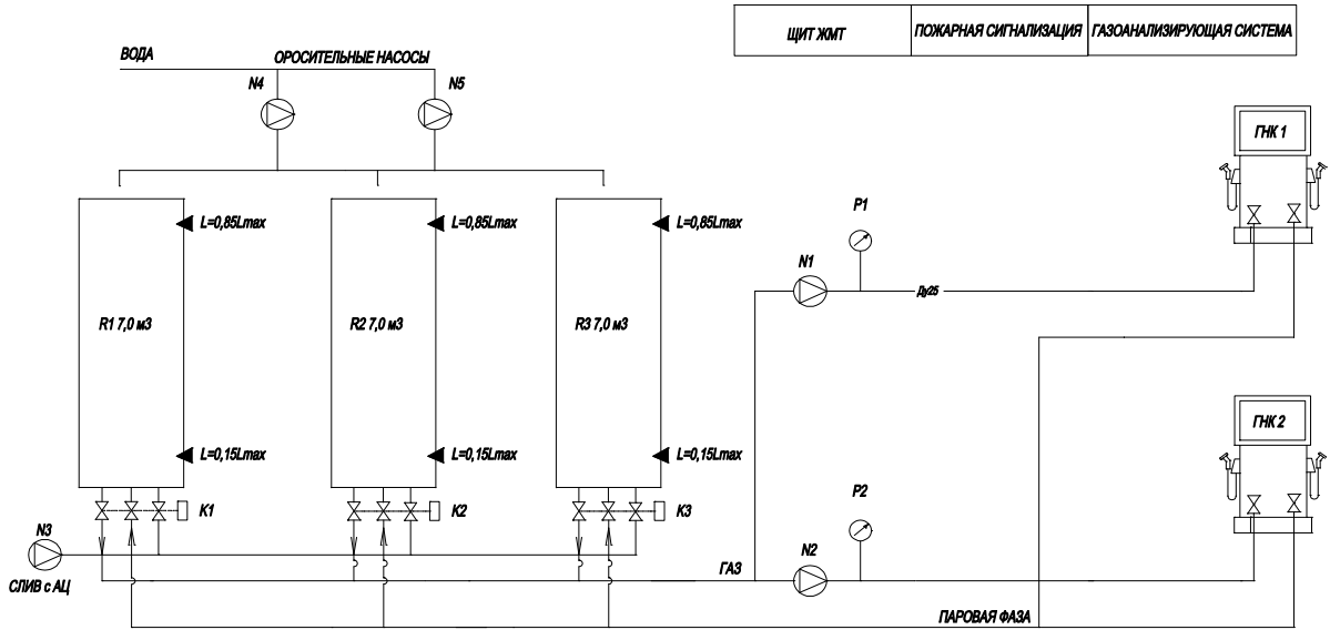
Технологическая схема АГЭС с отдельными (на резервуар) клапанами.
