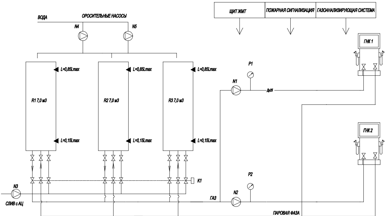
Технологическая схема АГЭС с общим (на все резервуары) клапаном.
