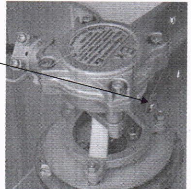
б) с измерителем объема СУГ
