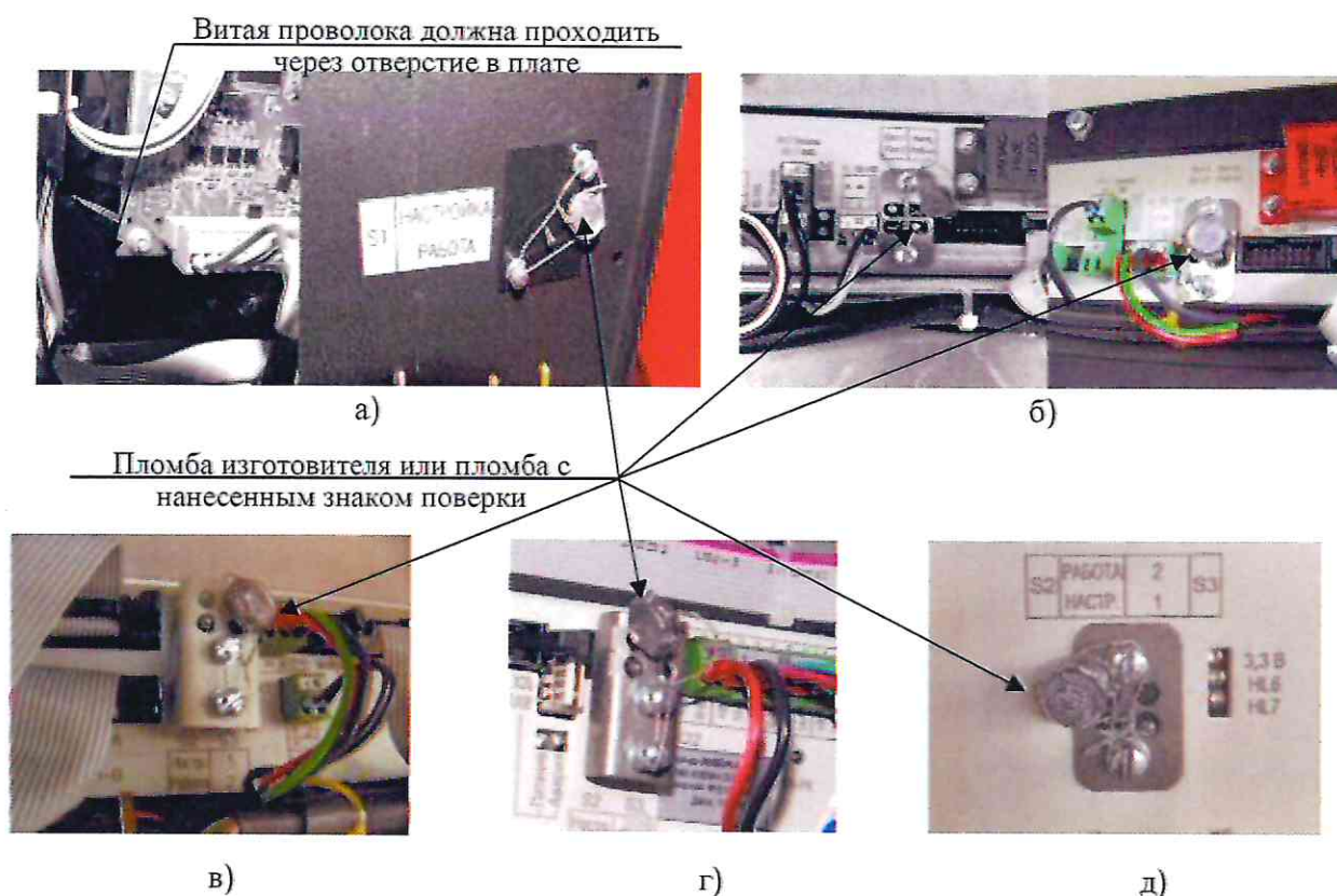
Рисунок 16 – Схемы пломбировки блоков управления серии «Топаз-306БУ» Примечание ¼ В блоках управления с параметром «Калибровочный код» тумблер «Работа/настройка» пломбируется собственными пломбами службы безопасности.
