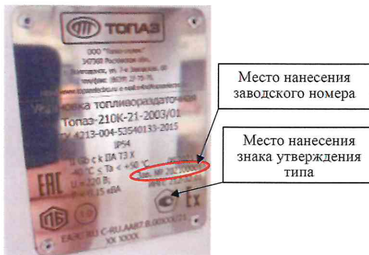
Рисунок 17 – Маркировочная табличка
