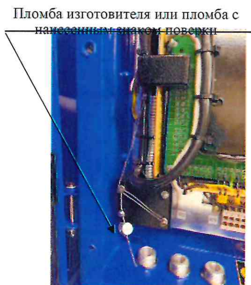
Рисунок 14 – Схема пломбировки устройства приема и обработки сигналов «Топаз-273Е»
