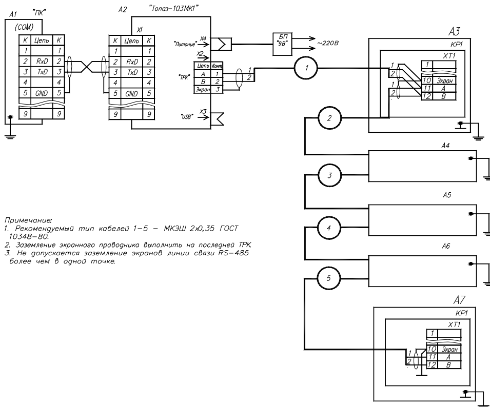
Рисунок Д.2 Линия связи "RS-485" для АЗС с УТ "ТОПАЗ"
