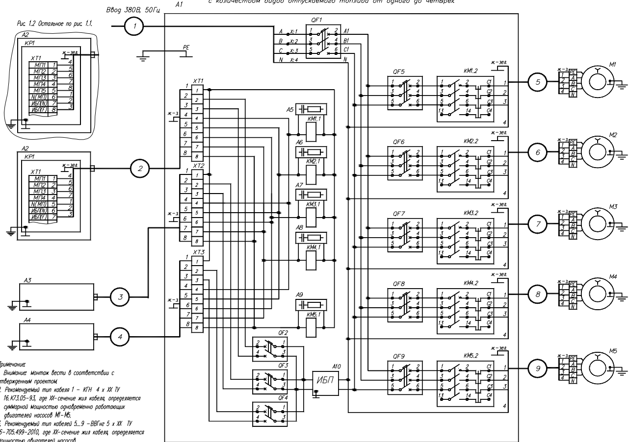
Рис. 1.1 Схема электрическая подключения силовой части напорных ТРК (УТ) с количеством вводов отпущаемого топлива от одного до четырех
