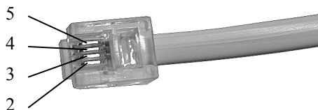
Нумерация контактов вилки 6P4С (контакты 1 и 6 отсутствуют)
