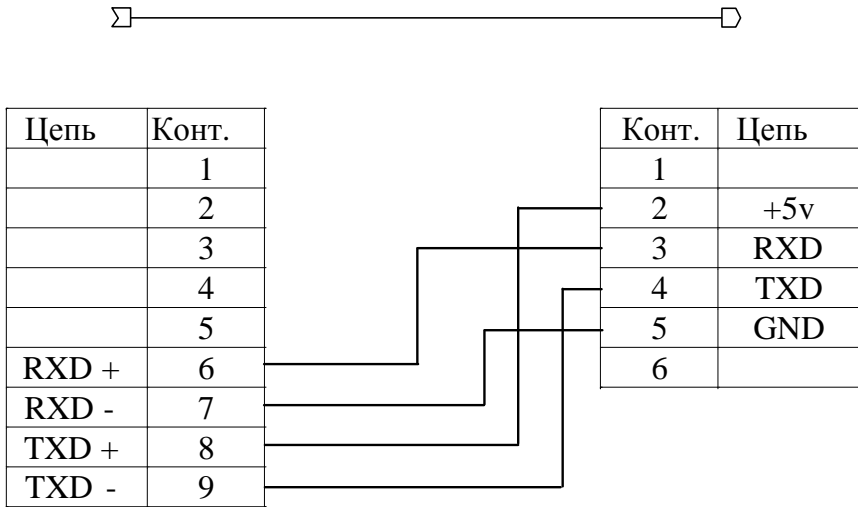
Рисунок Ж.2 - Схема кабеля K23
