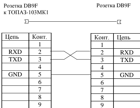
Рисунок Г.2 – Схема кабеля К21
