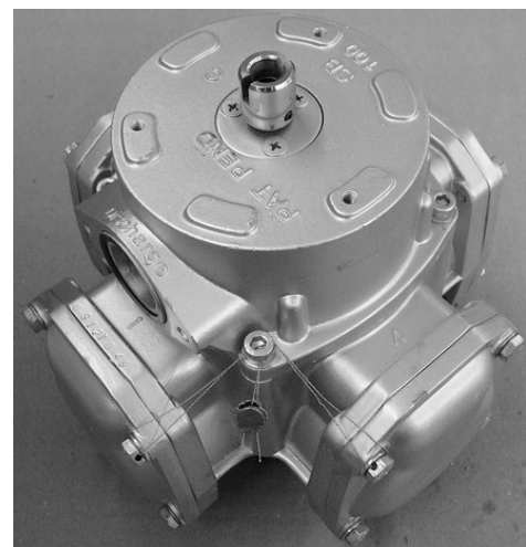
Рисунок Г.3 Пломбировка измерителя объёма
