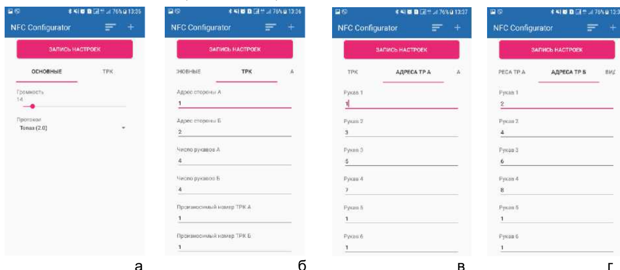
Рис. В.3 Запись настроек, конфигурация УТ
