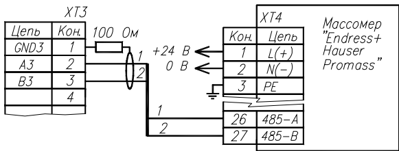
Рисунок 6. Подключение к расходомеру "Endress+Hauser Promass".
