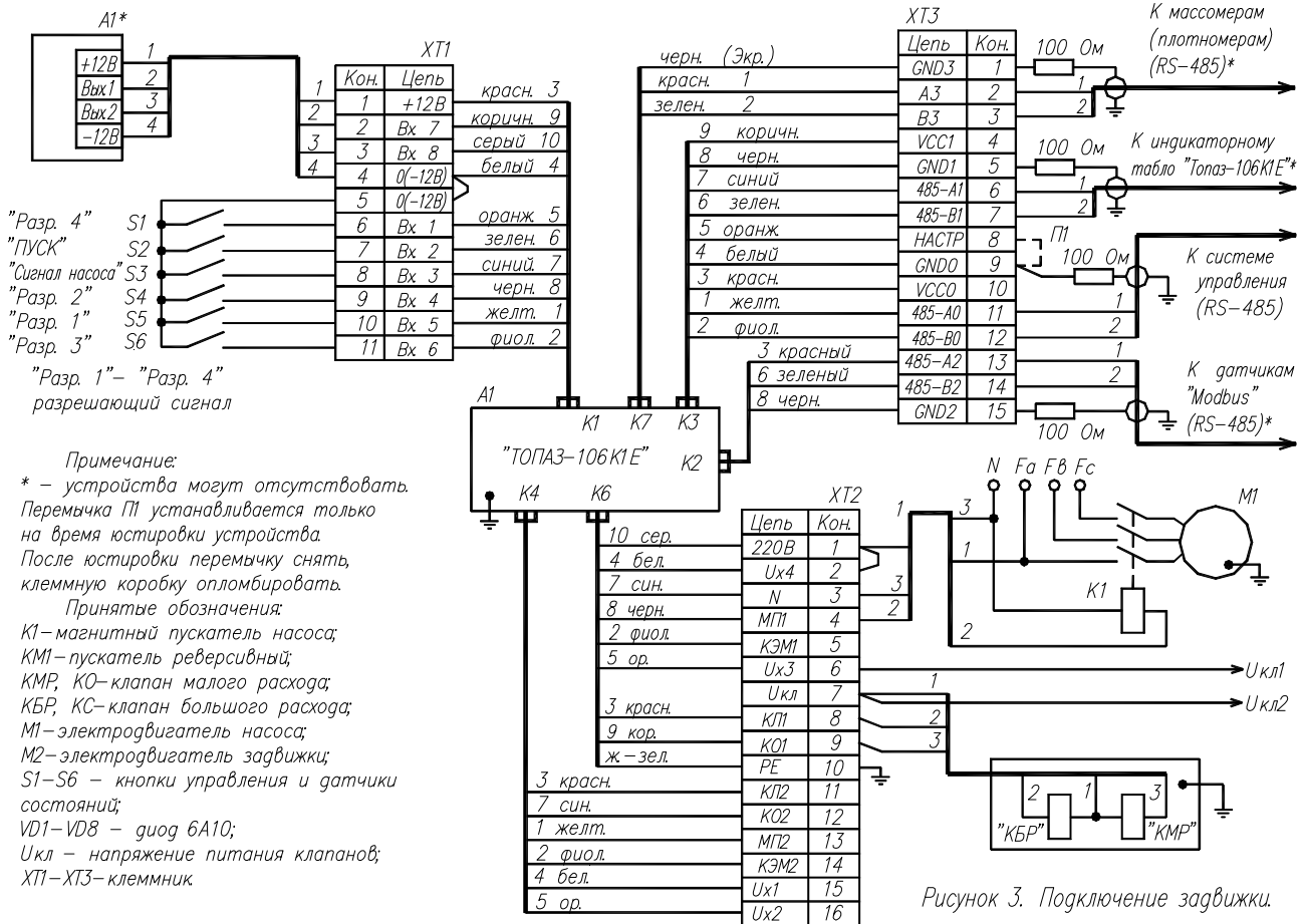
Рисунок 1. Схема электрическая подключения отсчетного устройства "Топаз-106К1Е" к измерительной установке. (Варианты подключения к устройствам различных типов показаны на рисунках 2-8.)
