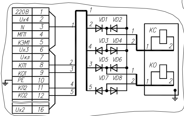
Рисунок 2. Подключение клапанов 110 В постоянного тока. Остальное по рисунку 1.
