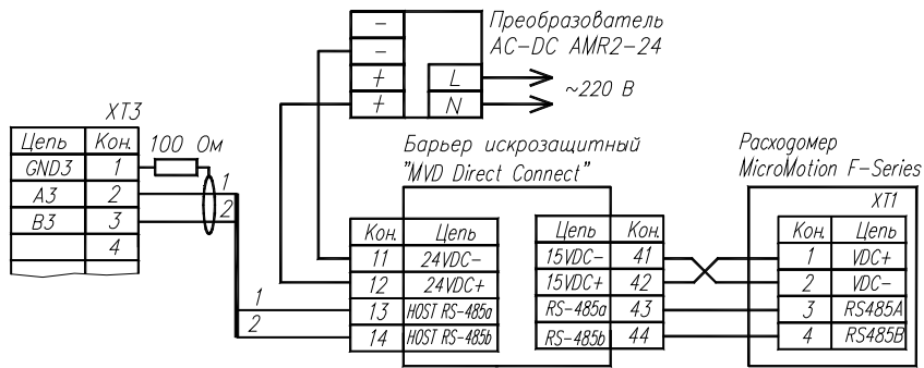
Рисунок 4. Подключение к расходомеру MicroMotion.
