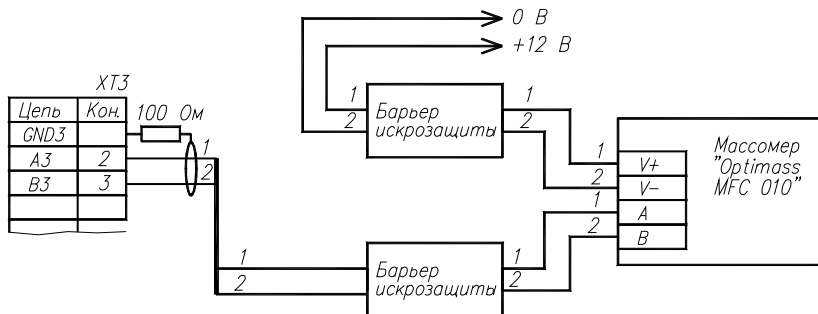
Рисунок 8. Подключение к расходомеру "Optimass MFC 010".
