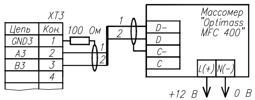
Рисунок 7. Подключение к расходомеру "Optimass MFC 400".
