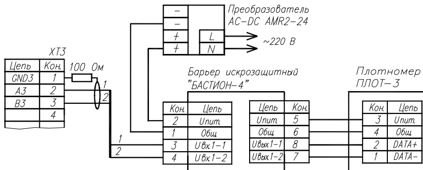
Рисунок 5. Подключение к плотномеру ПЛОТ-3.
