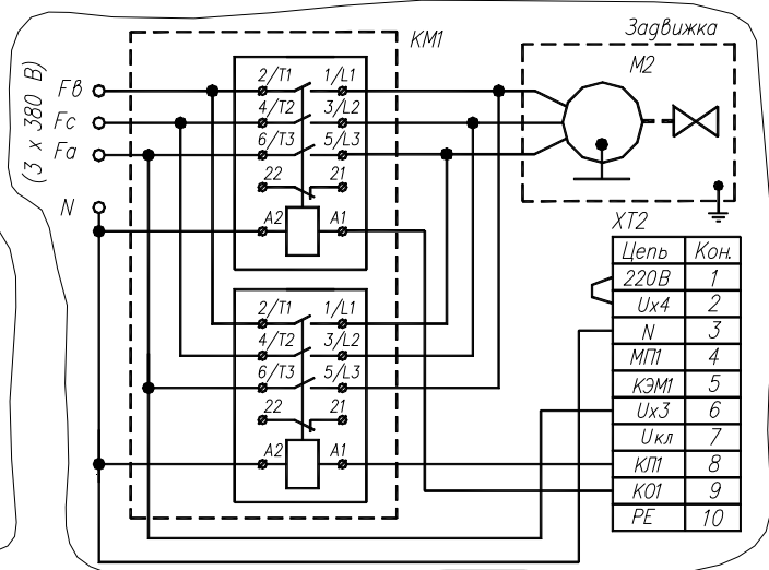
Рисунок 3. Подключение задвижки.
