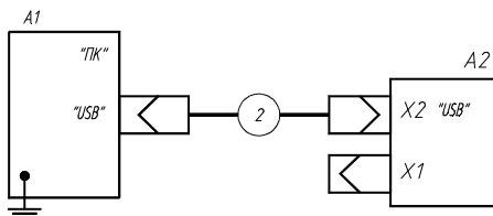
Рис. 3. Подключение счетчика к персональному компьютеру.
