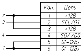
Розетка IDC-06F
