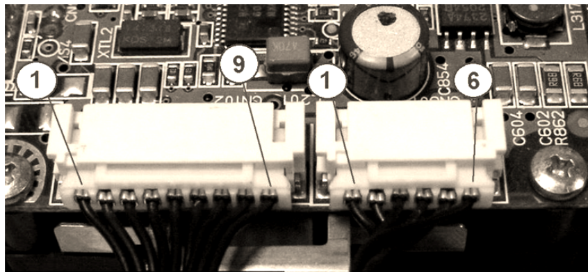
Цоколевка разъемов картридера (A17).
