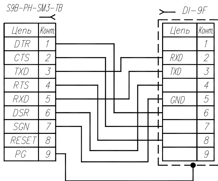
Схема кабеля 6.4
