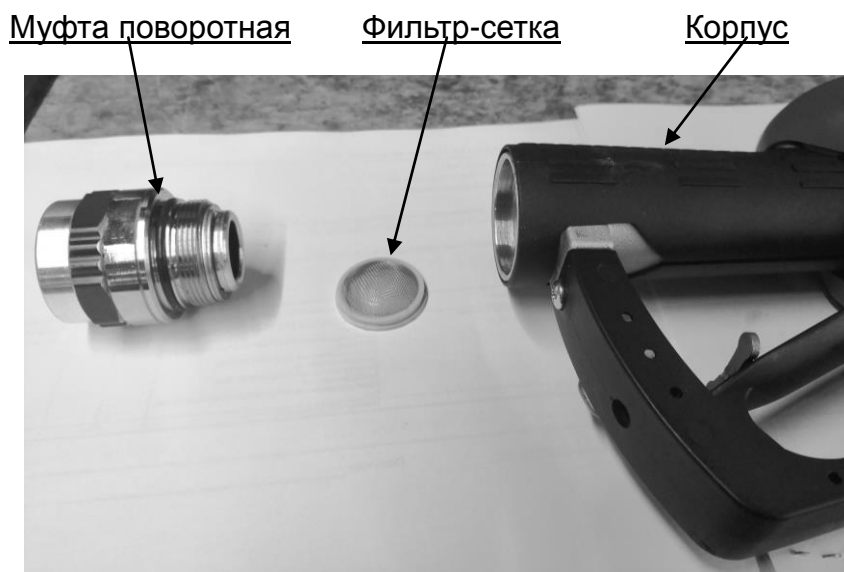
Рисунок 9 — Расположение фильтр-сетки в раздаточном кране
